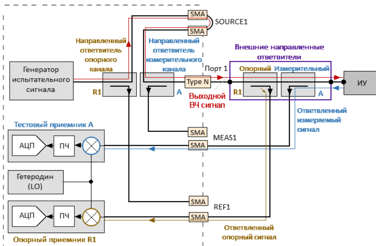
Рисунок 232 – Анализатор C2209, распространение сигнала в режиме прямого доступа
