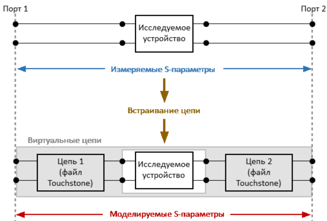
Рисунок 196 – Встраивание цепи
