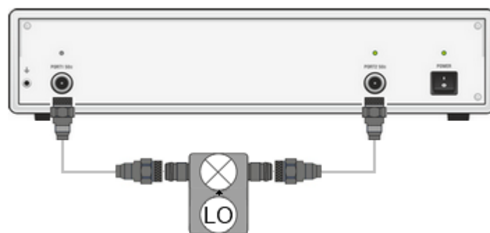
Рисунок 219 — Измерение смесителя со встроенным гетеродином (синхронизация невозможна)
