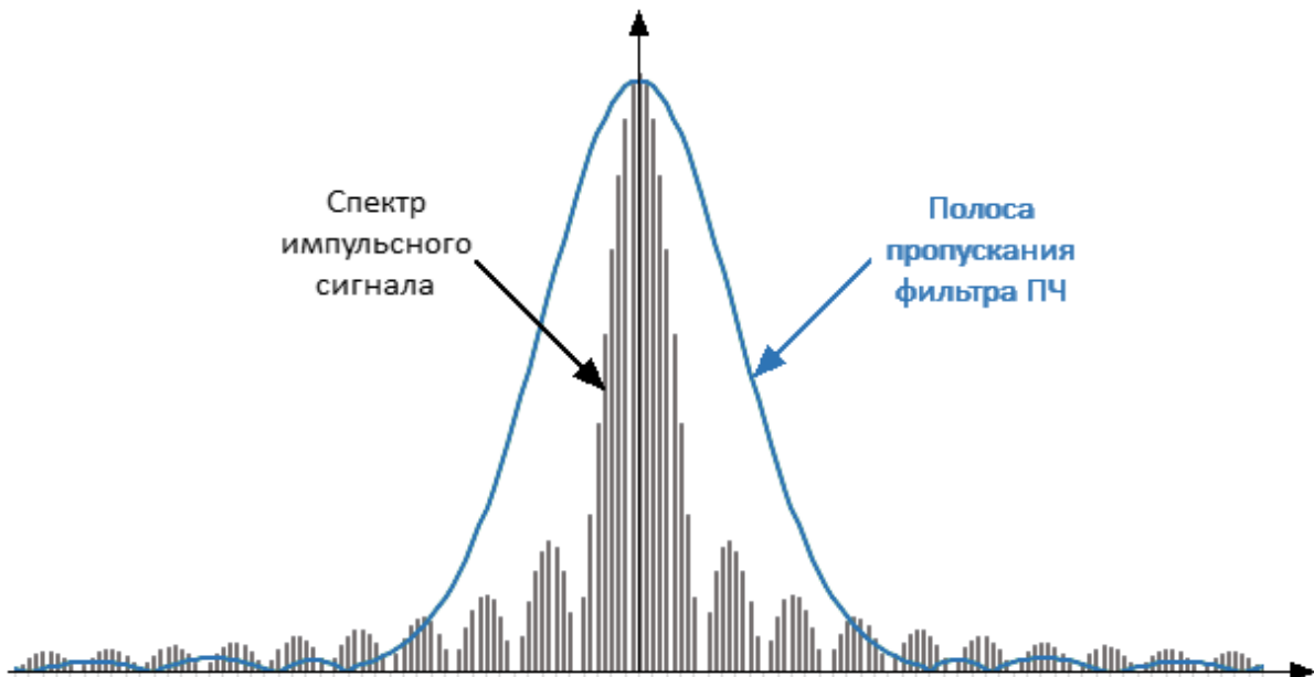
Рисунок 248 – Широкополосное детектирование
