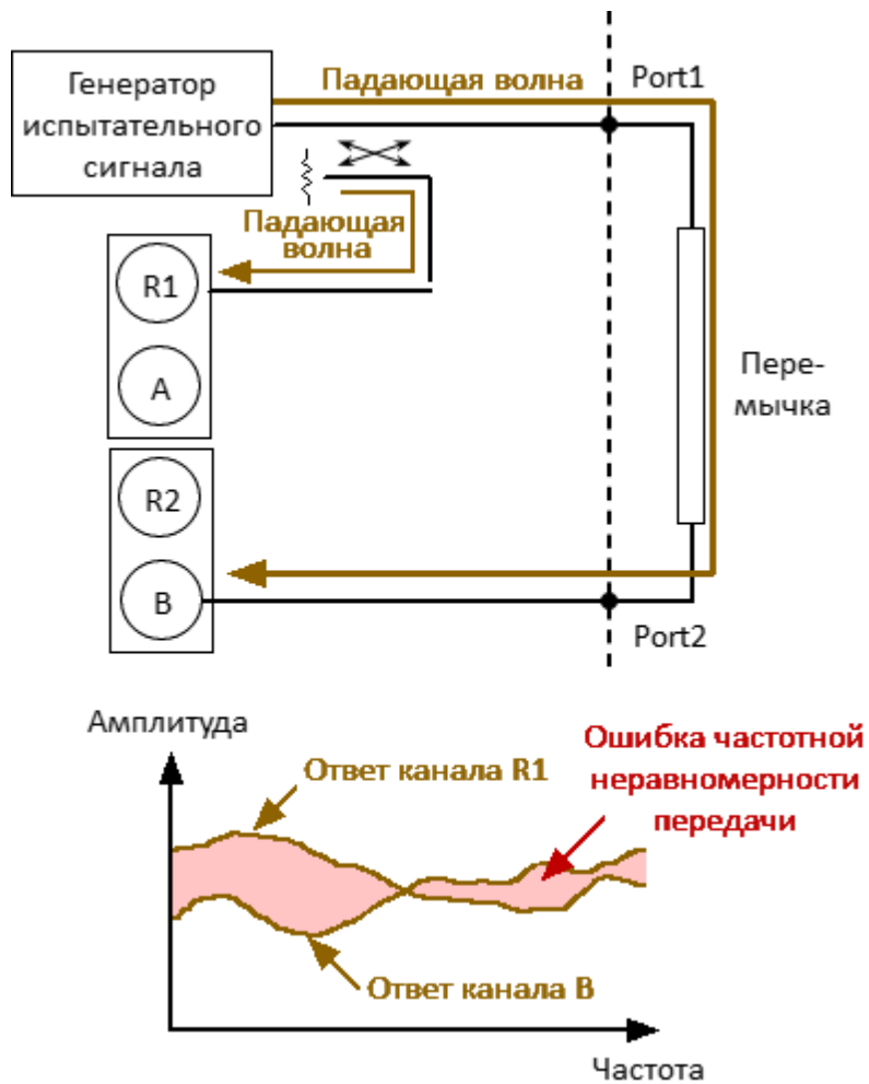
Рисунок 116 – Ошибка частотной неравномерности передачи
