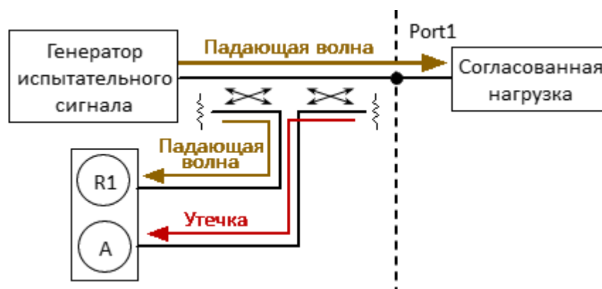
Рисунок 112 – Ошибка направленности
