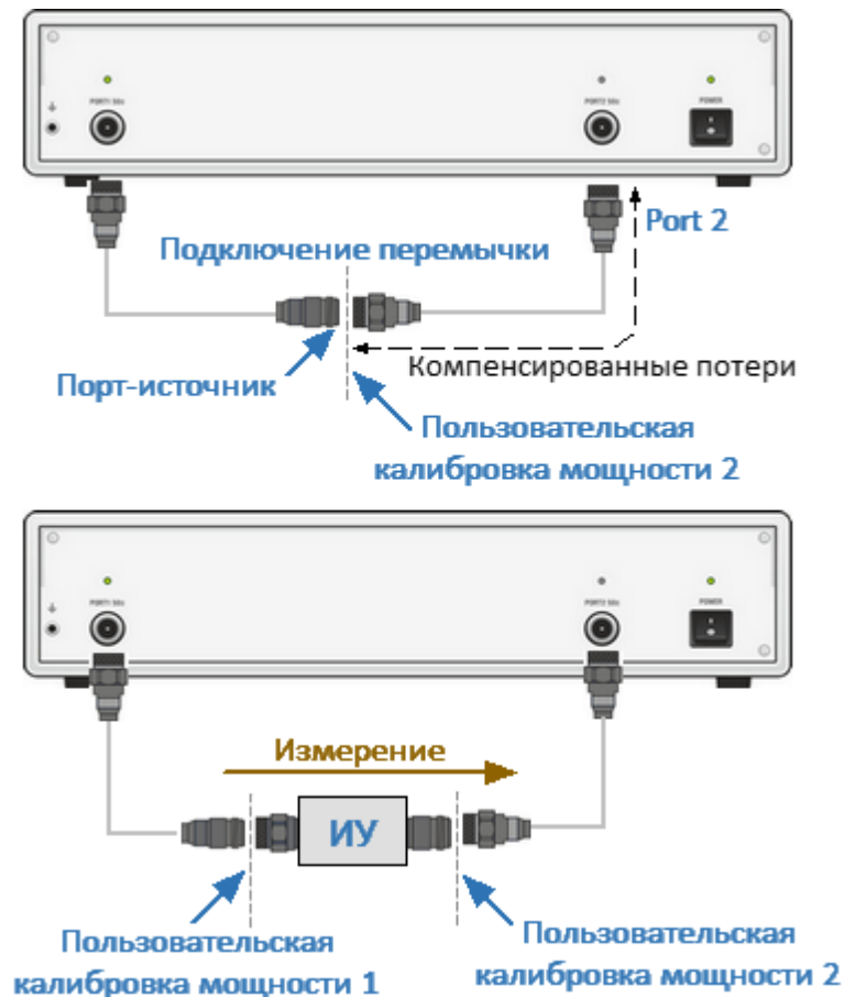
Рисунок 155 – Калибровка приемников
