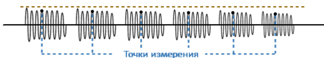
Рисунок 261 – Пример изменения коэффициента усиления от импульса к импульсу
