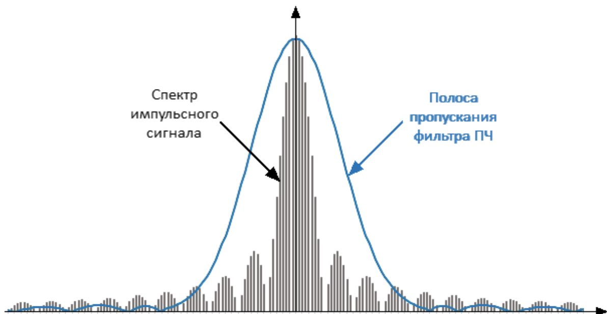
Рисунок 238 – Широкополосное детектирование
