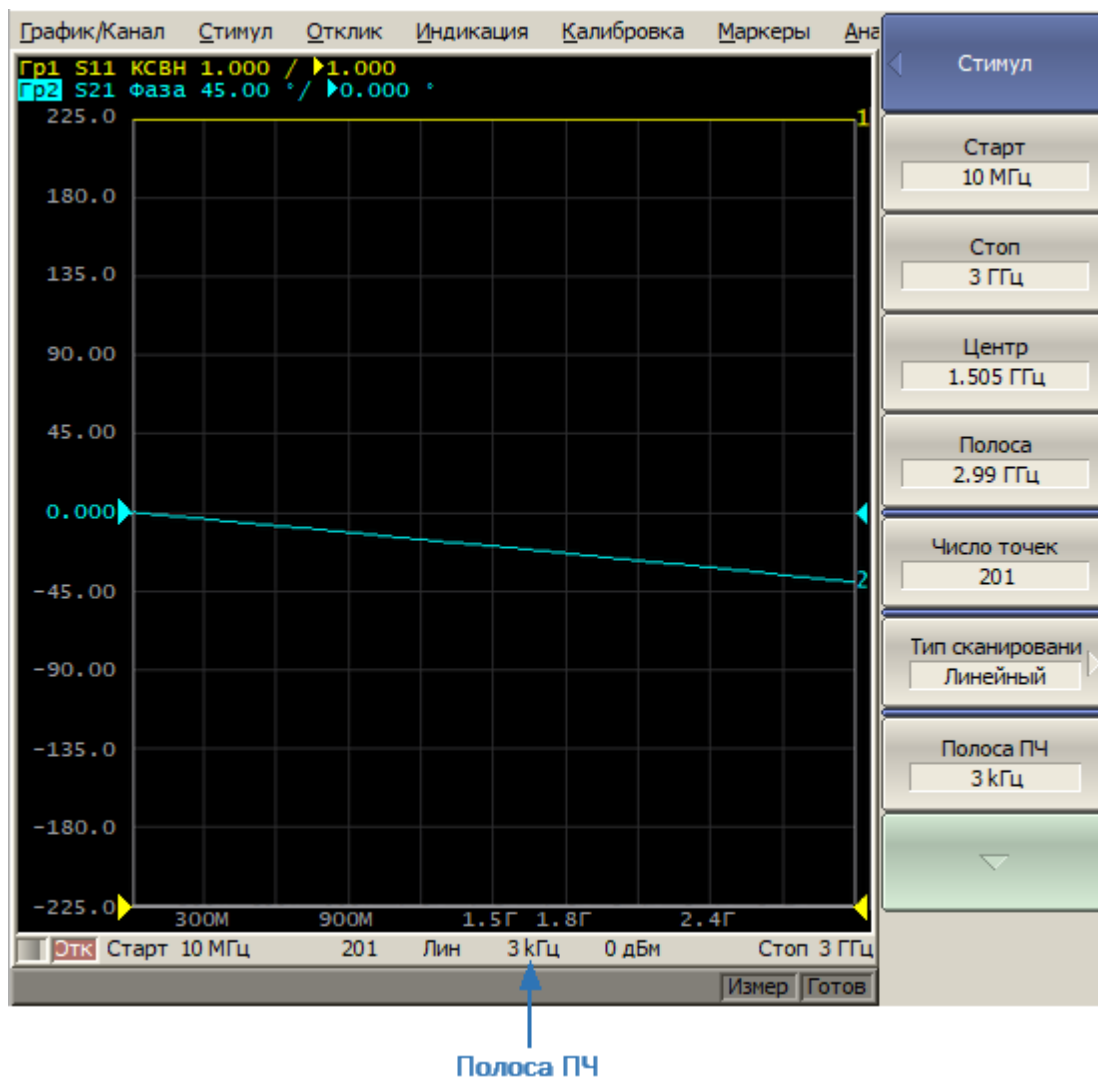
Рисунок 42 – Полоса пропускания ПЧ в строке состояния канала
